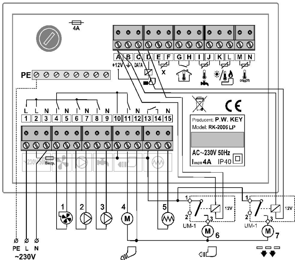
Рис. 2. Диаграмма подключения контроллера RK-2006LP.
